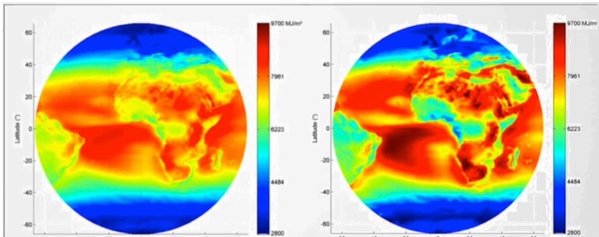
Moyenne sur 2004-2010 de l'irradiation annuelle globale horizontale (gauche) et directe en incidence normale (droite) issue de la base de données HelioClim-3 (méthode Heliosat-2) créées par MINES ParisTech ( www.soda-is.com )
